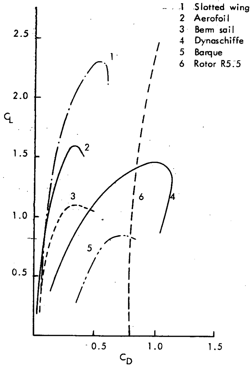
FIG.3. SAIL POLAR DIAGRAM.
