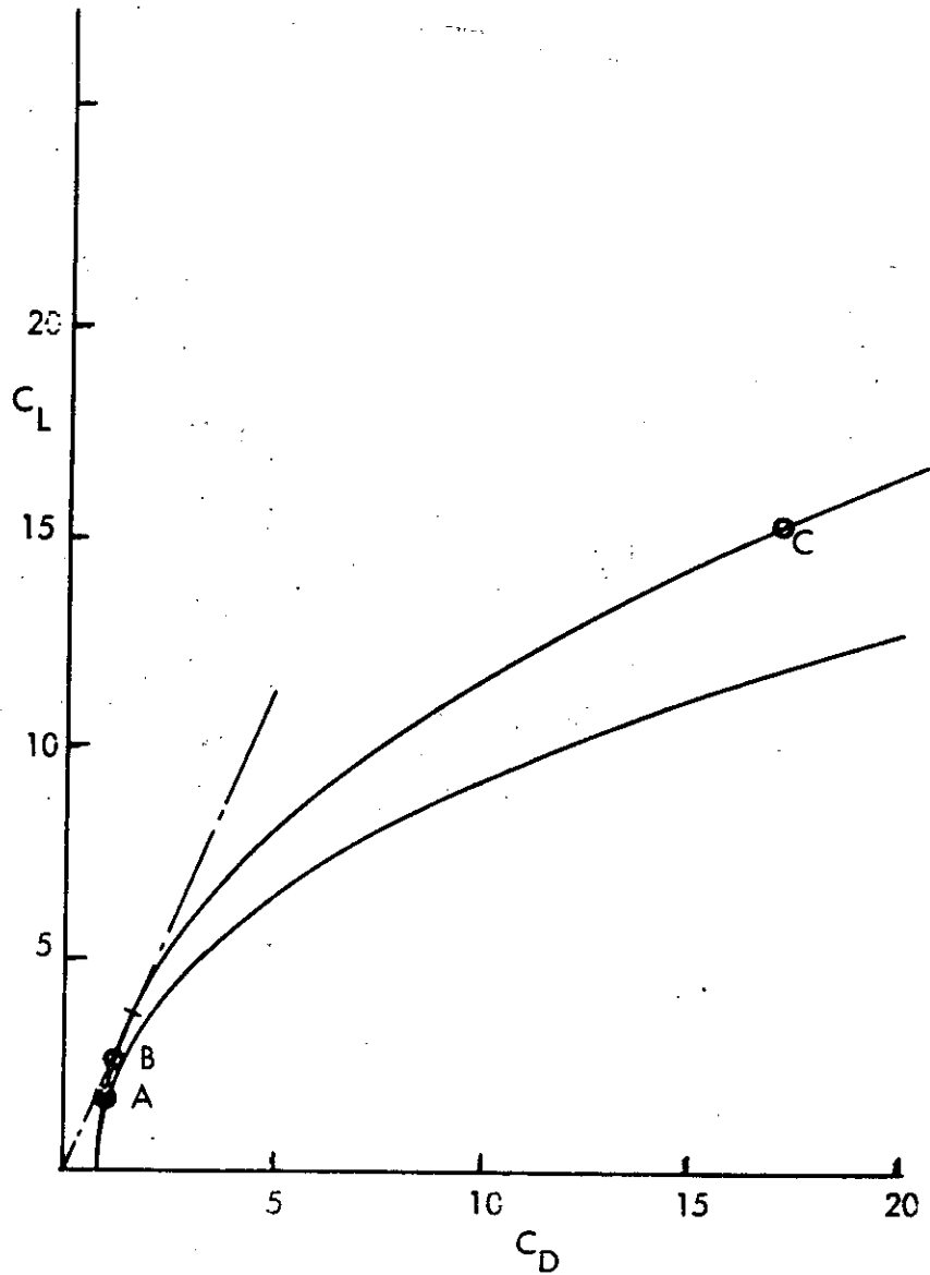
FIG.4. FLETTNER ROTOR.
